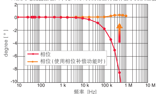
AC/DC电流直接输入单元PW9100的相位特性补偿示例(典型值)
